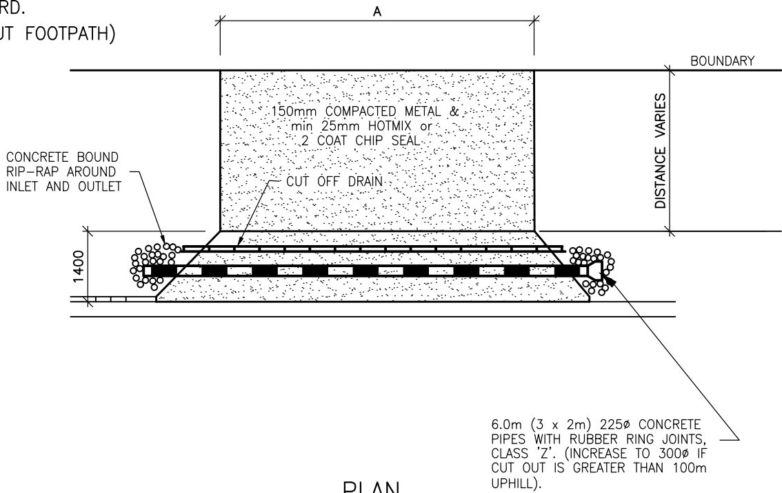
PLAN N.T.S.
